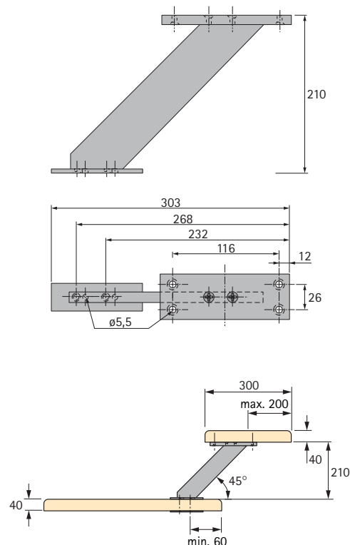
Barová konzola výšky 210 mm
