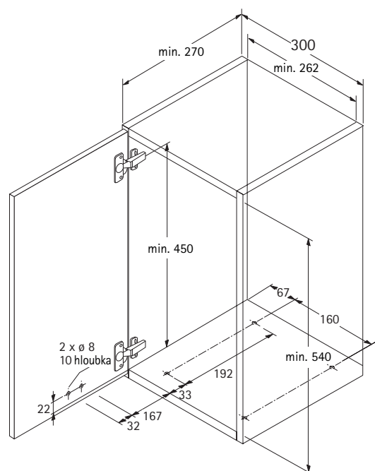
Rozměry korpusu a vrtání pro skříňku šířky 300 mm
