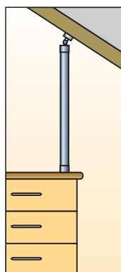
Osová trubka a adaptér pro šikmé stropy, od pracovní desky až po šikmý strop.
