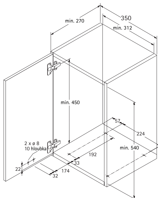
Rozměry korpusu a vrtání pro skříňku šířky 350 mm
