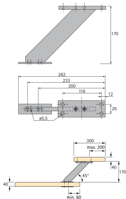
Barová konzola výšky 170 mm
